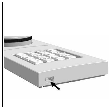
Abbildung 2: Mini-USB Buchse Sonderschnittstelle, nur in Verbindung mit Original dormakaba CB90 PC-Kabel verwenden!
