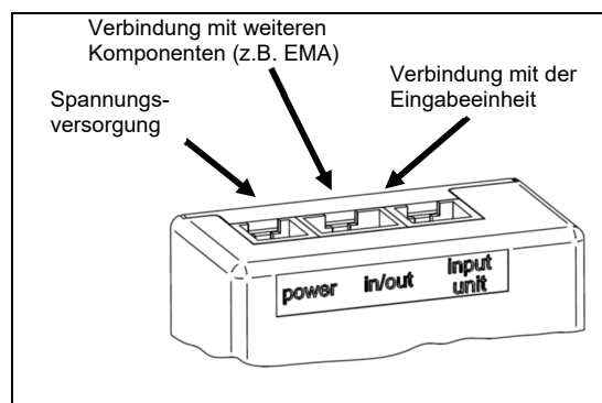
Abbildung 4: Anschlüsse am Schlossgehäuse
